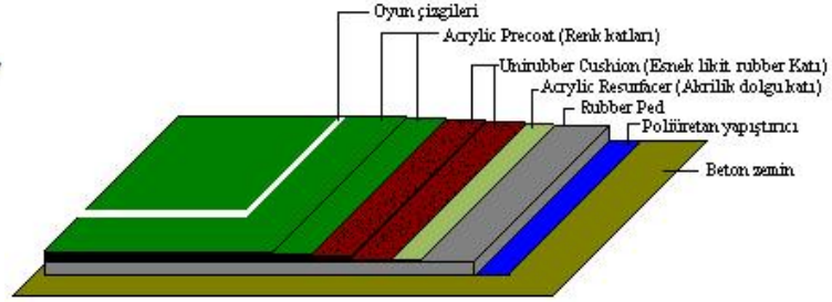
RUBBER ÜZERİ CUSHION KATMANLI AKRİLİK DETAYI
