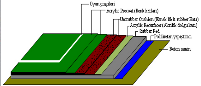
RUBBER ÜZERİ CUSHION KATMANLI AKRİLİK DETAYI
